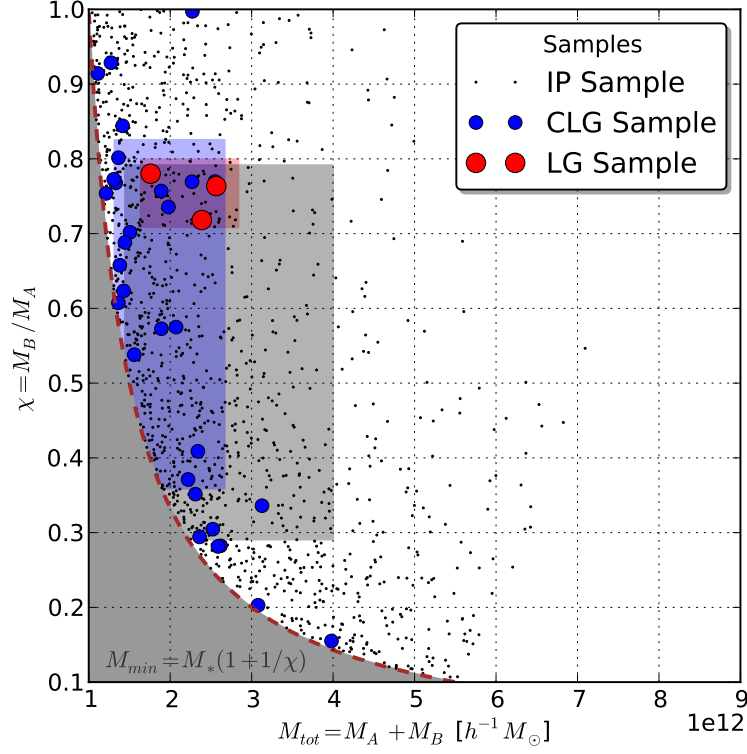
Figura 4.12: Diagrama de dispersión de los parámetros de masa definidos ( M_{tot}, \chi ) para cada una de las muestras de pares. Las regiones cuadradas son construidas a partir del valor medio y la desviación estándar de la muestra del mismo color. La región gris en la parte inferior izquierda corresponde a un corte impuesto artificialmente con el rango mínimo de masa de los halos tomados M_* para construir las muestras de pares.
