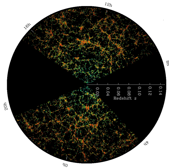
Figura 1.5: Mapa del universo a gran escala de acuerdo al Sloan Digital Sky Survey. Tomado de la página oficial del proyecto http://www.sdss.org/
