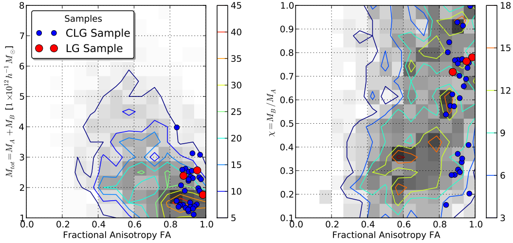
Figura 4.13: Diagramas de dispersión para el fraccional de anisotropía respecto a los parámetros de masa. El mapa de fondo y las curvas de contorno corresponden a número de pares de la muestra IP .
