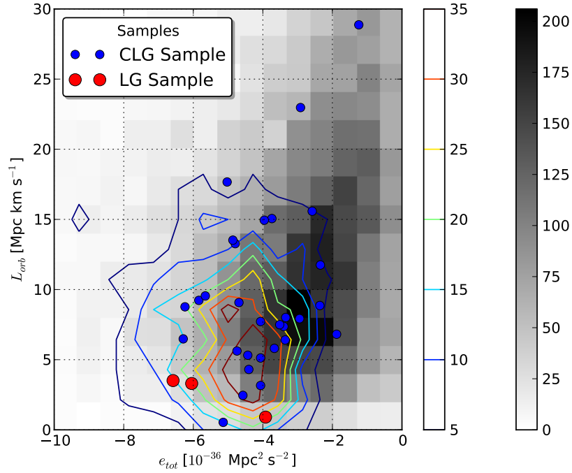
Figura 4.14: Diagrama de dispersión para la energía total y el momentum angular orbital de los sistemas de pares. El mapa de fondo corresponde a la distribución de la muestra P , mientras las líneas de contorno a la distribución de la muestra IP , en ambos casos los valores corresponden al número de pares.
