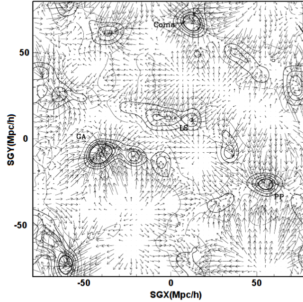
Figura 3.6: Campo de densidad y campo de velocidad peculiar inicial contruidos a partir de restricciones para la reproducción del entorno local en una escala de 160 h^{-1} \text{Mpc} . Algunas estructuras identificadas son: Coma , cúmulo de coma, PP , supercúmulo de Perseus-Pisces, LS , supercúmulo local, GA , gran atractor. La flecha superior derecha indica la escala del campo de velocidad peculiar en 1000 km/s. Tomado de [22].
