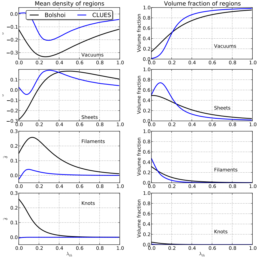
Figura 4.4: Parámetro de densidad medio para diferentes tipos de regiones en función del valor umbral \lambda_{th} (paneles izquierda). Fracciones de volumen normalizadas para diferentes tipos de regiones, también acorde al valor umbral \lambda_{th} .
