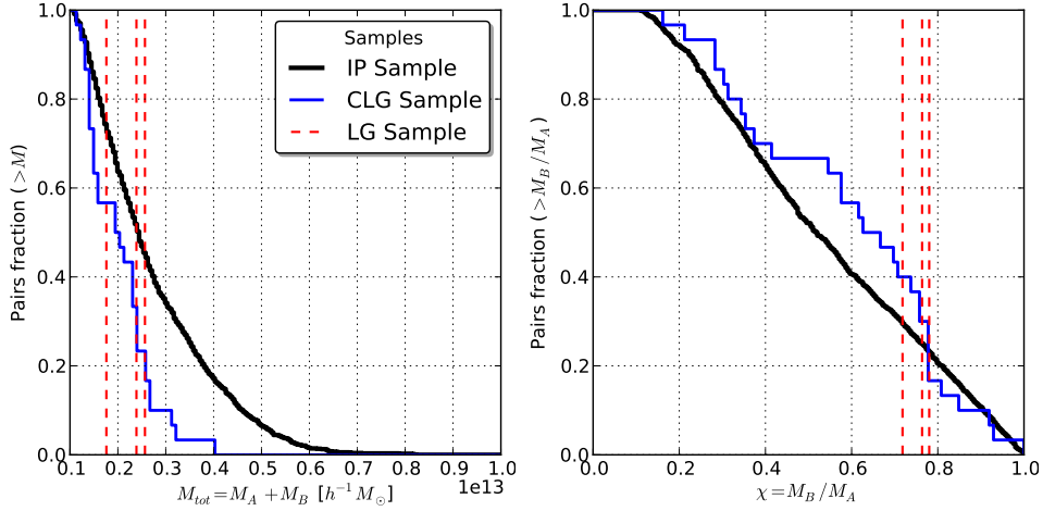
Figura 4.11: Funciones de distribución integrada para la masa total M_A + M_B (izquierda) y la razón de las masas M_B/M_A (derecha), de las muestras de pares en Bolshoi.
