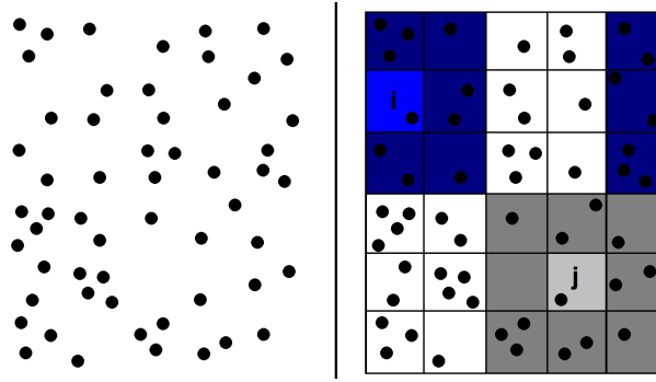
Figura 3.14: Ilustración 2D del método para la detección de las muestras de pares. Distribución de halos de materia oscura (izquierda), definición de zonas (derecha).
