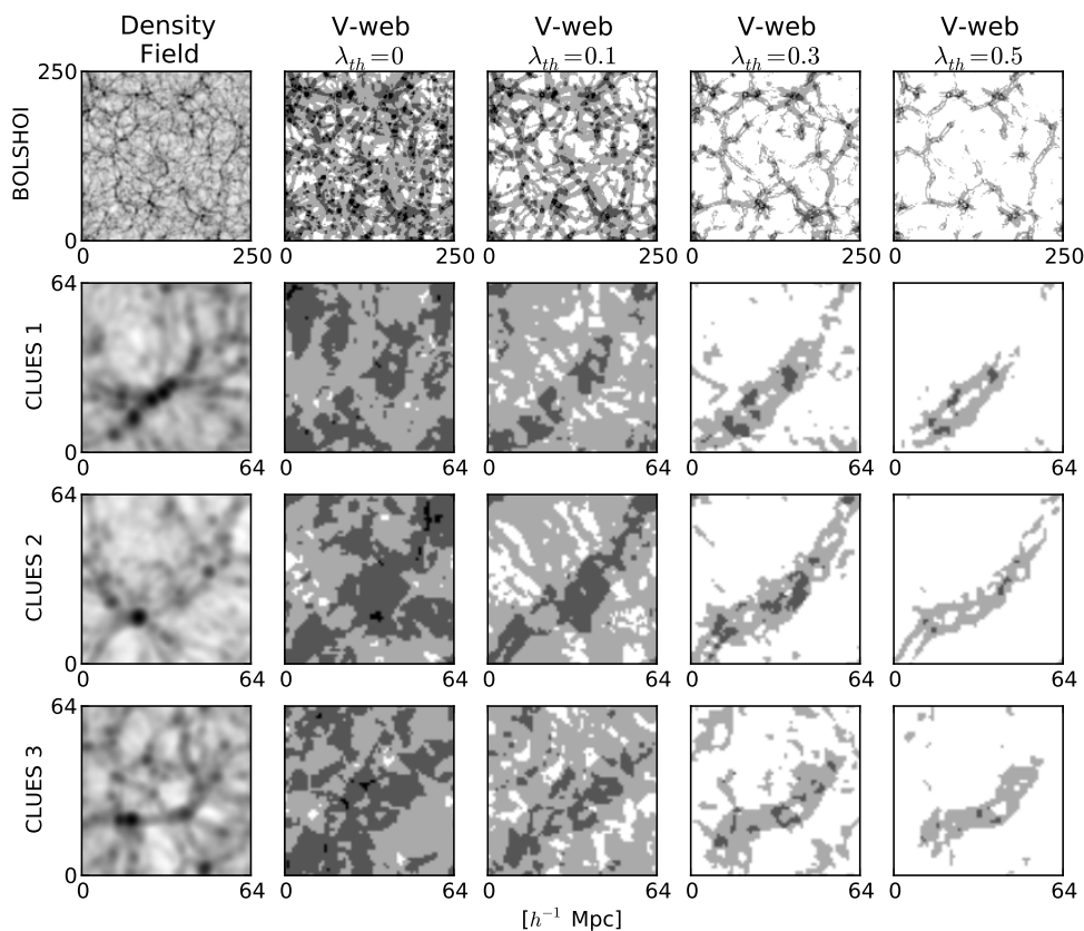
Figura 4.5: Comparación de la impresión visual obtenida con el método V-web para varios valores del parámetro \lambda_{th} . Se usa el siguiente esquema de clasificación (Negro - Nudo, Gris oscuro - Filamento, Gris - Hoja, Blanco - Vacío). La resolución de cada malla es 1,0h^{-1} Mpc/celda, con un suavizado Gaussiano de una celda. El grosor de cada slide es de una celda.
