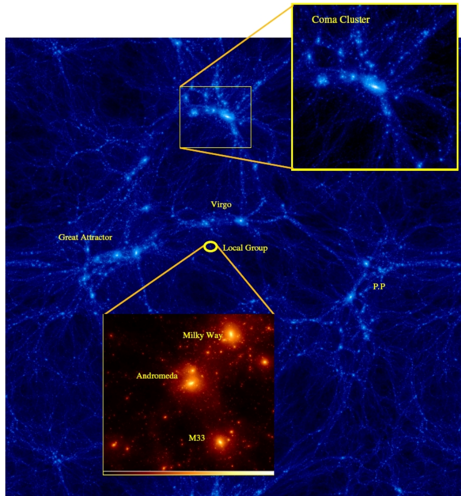
Figura 3.8: Simulación obtenida en el proyecto CLUES. En esta se muestran las estructuras a gran escala del universo local y se aprecian con claridad los miembros más significativos del grupo local. Tomado de la página oficial del proyecto http://www.clues-project.org
