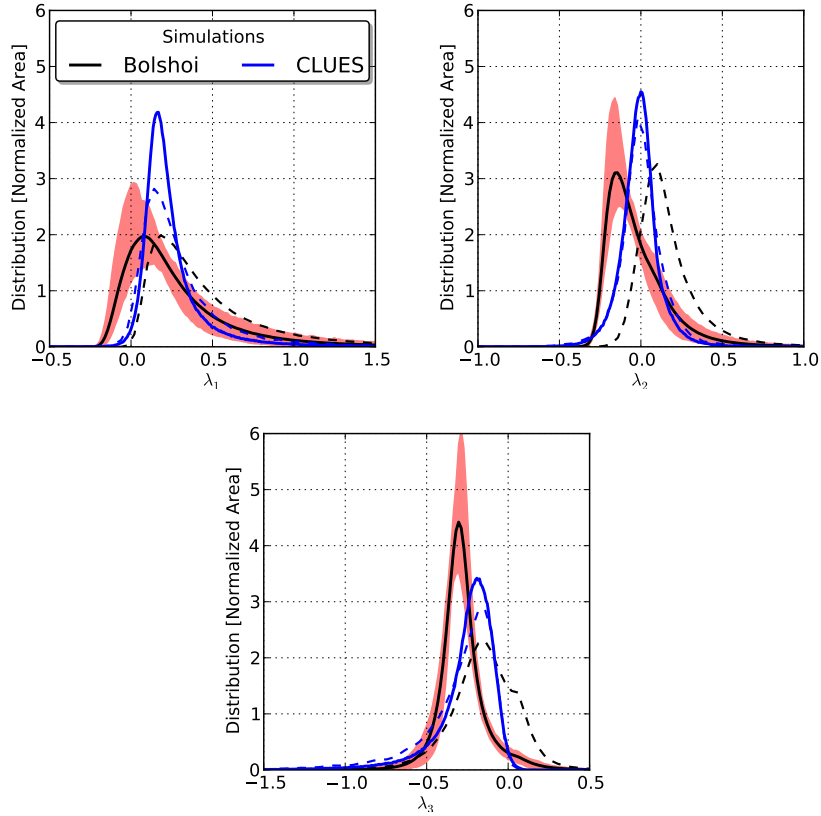
Figura 4.3: Distribución de los autovalores en el esquema V-web para cada una de las celdas de volumen (línea continua) y para los entornos de los halos de materia oscura en los catálogos FOF (línea discontinua). Las distribuciones están normalizadas tal que su área es la unidad. Resolución de 1,0h^{-1} Mpc/celda y suavizado Gaussiano de una celda.
