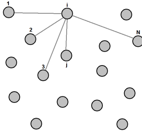
Figura 3.1: Formulación del problema de N-cuerpos.
