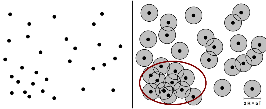
Figura 3.11: Diagrama ilustrativo del método FOF. Los círculos grises entorno a cada partícula representa la zona de vinculación y la curva roja representa una de las estructuras encontradas.
