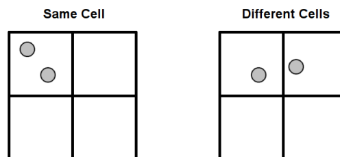
Figura 4.6: Situación patológica respecto al entorno de los sistemas de pares de halos.
