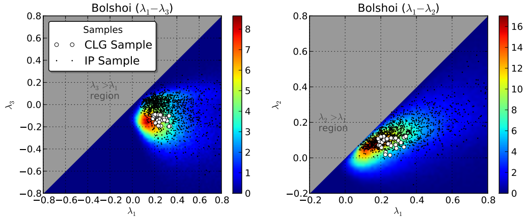
Figura 4.8: Distribuciones 2D del entorno cosmológico para diferentes muestras, \lambda_1 - \lambda_3 (izquierda) y \lambda_1 - \lambda_2 (derecha). El histograma de fondo, graficado en colores, corresponde a la distribución de entorno para todos los halos de Bolshoi (muestra GH ), su resolución es de 100 \times 100 para el rango mostrado y están normalizados respecto a su área. Los puntos negros corresponden a la distribución de la muestra IP y finalmente los puntos blancos a la muestra CLG .
