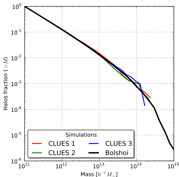
Figura 4.2: Funciones de masa integrada de halos de materia oscura (muestra GH) para cada simulación.
