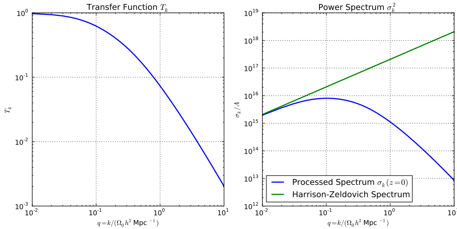
Figura 2.7: Función de transferencia para materia oscura fría en la época actual [26] (Izquierda). Comparación entre el espectro de potencia inicial, Harrison-Zeldovich, y el espectro de potencia procesado (derecha).
