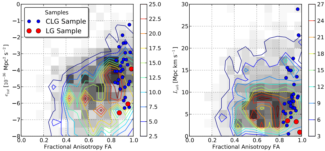
Figura 4.15: Diagramas de dispersión para el fraccional de anisotropía respecto a la energía y el momentum angular. El mapa de fondo y las curvas de contorno corresponden a número de pares de la muestra IP .
