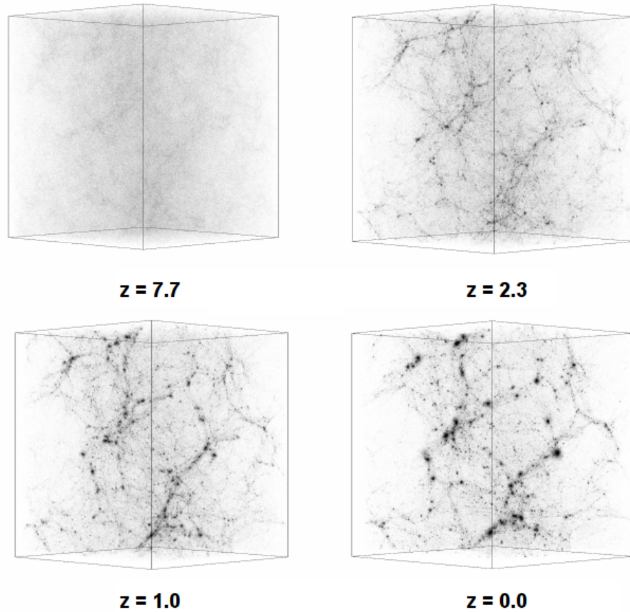
Figura 2.8: Evolución de una simulación numérica de materia oscura en una caja de 40 Mpc/h, iniciando en un estado de alta homogeneidad (arriba-izquierda) hasta la época actual de estructuras altamente no lineales (abajo-derecha). Tomado de http://www.astro.utu.fi/research/CosmoS/lss/lss_p1.shtml
