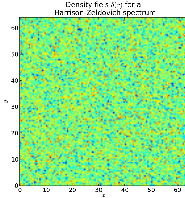
Figura 2.6: Distribución inicial de perturbaciones para el campo de contraste de densidad a partir de la distribución Gaussiana 2.57 y el espectro de potencia de Harrison-Zeldovich \sigma_k \propto k .
