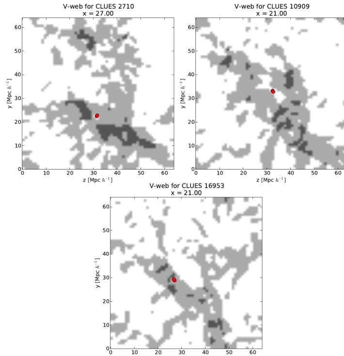
Figura 3.13: Entorno cosmológico a partir del esquema V-web (con \lambda_{th} = 0,3 ) para cada uno de los LG de las simulaciones CLUES, indicados por los puntos rojos.
