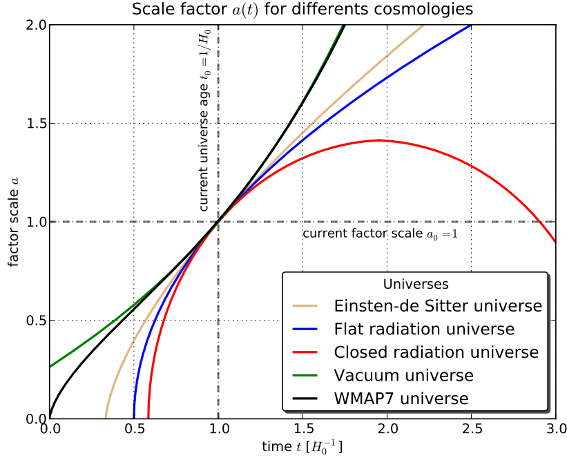
Figura 2.3: Diferentes soluciones de universo para las ecuaciones de Friedmann.
