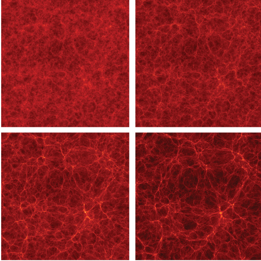
Figura 3.5: Evolución de la simulación Bolshoi. Se ilustran el campo de densidad de una región rectangular de 16 \text{ Mpc}/h de grosor y 250 \text{ Mpc}/h de lado para diferentes estadios de evolución. z = 9,5 (superior izquierda), z = 3 (superior derecha), z = 1 (inferior izquierda) y z = 0 (inferior derecha). Tomado de http://spectrum.ieee.org/aerospace/astrophysics/the-cosmological-supercomputer
