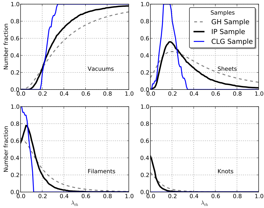
Figura 4.9: Fracciones de cantidad de objetos en diferentes regiones en función del valor umbral \lambda_{th} . Para el caso de la muestra GH se cuentan número de Halos, mientras que para las muestras IP y CLG número de pares.
