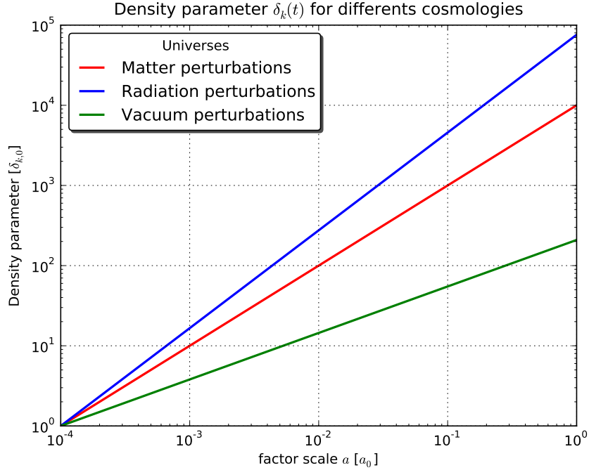
Figura 2.5: Evolución de los modos normales del campo de densidad. Por motivos ilustrativos se ha normalizado respecto a las condiciones iniciales.
