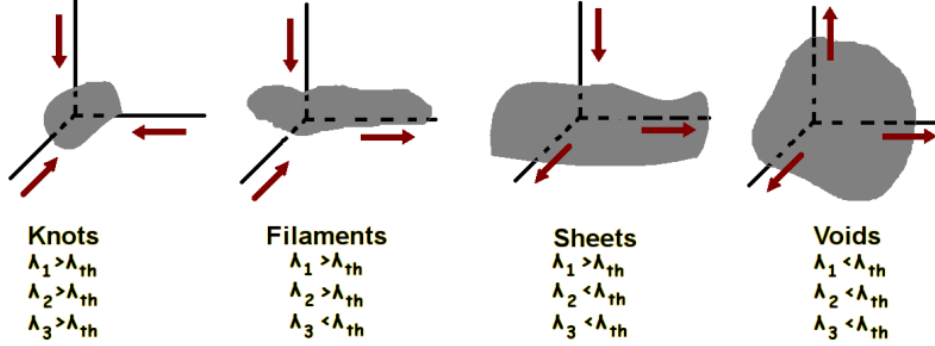
Figura 3.9: Esquema de clasificación del entorno cosmológico para los esquemas T-web y V-web. El valor umbral \lambda_{th} es tomado como un parámetro libre.
