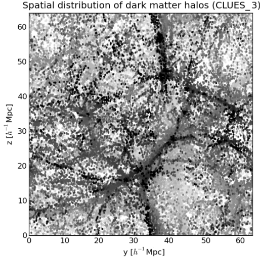
Figura 3.12: Halos encontrados a partir del esquema FOF en una de las simulaciones CLUES. El gradiente de color indica la profundidad respecto al eje x , donde los halos negros son los más cercanos.
