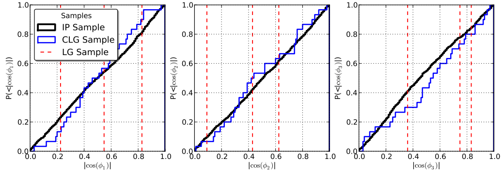
Figura 4.16: Histogramas integrados para el ángulo formado entre el momentum angular de los pares, el cual determina el plano orbital, y cada uno de los autovectores definidos por la V-web en el entorno cosmológico. Se realiza para cada las muestras de pares CLG y IP , mientras que los grupos locales de CLUES son ilustrados con las líneas rojas punteadas.
