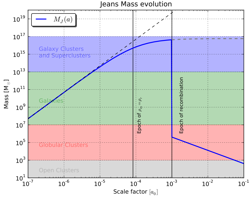
Figura 2.4: Evolución de la masa de Jeans para diferentes estadios del universo. En las regiones coloreadas se ilustra el rango típico de masa para varios tipos de estructuras, desde cúmulos estelares abiertos hasta cúmulos y supercúmulos de galaxias.
