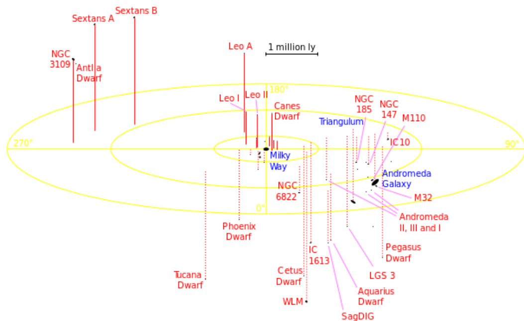
Figura 1.4: Grupo Local. Tomado de http://commons.wikimedia.org/wiki/File:Local_Group.svg
