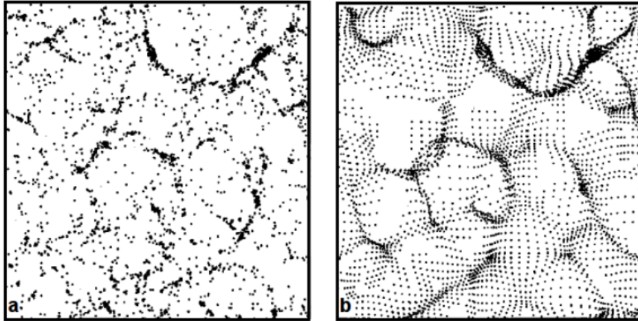
Figura 2.9: Comparación de la evolución en régimen no lineal entre una simulación de N-cuerpos (a), y la aproximación de Zeldovich (b). En ambos casos se usan las mismas condiciones iniciales. Tomado de [26].
