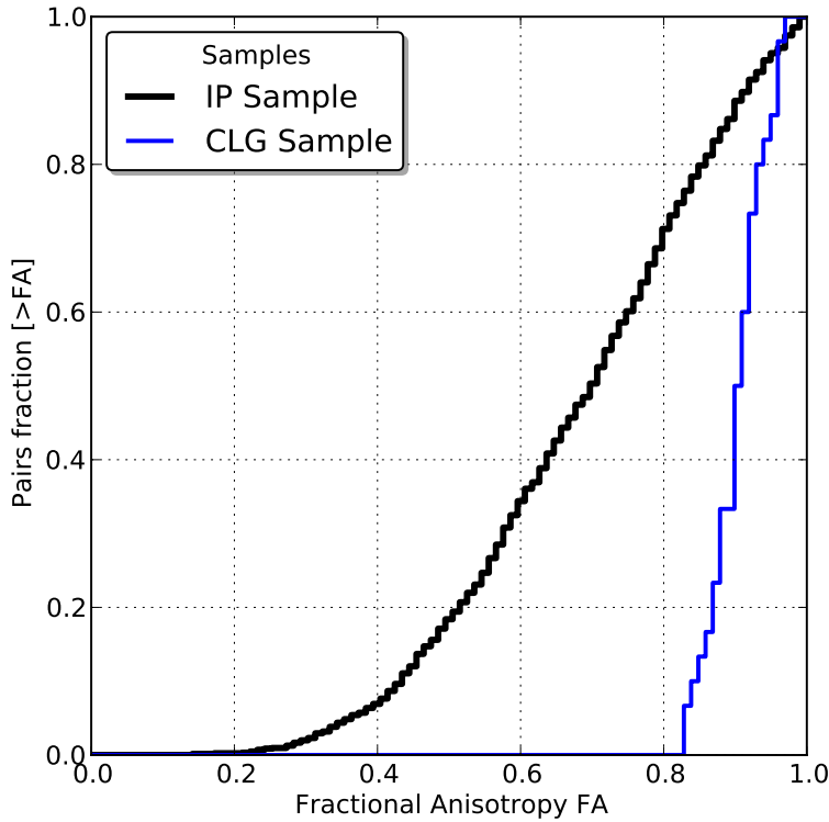
Figura 4.10: Histograma integrado del fraccional de anisotropía para las muestras de pares IP y CLG .
