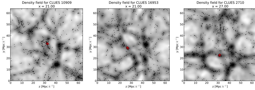
Figura 3.7: Tres simulaciones restringidas del proyecto CLUES en las se identifican sistemas tipo grupo local. Se ilustra el campo de densidad de cada simulación junto con los halos de materia oscura (puntos negros), y los grupos locales encontrados (puntos rojos).
