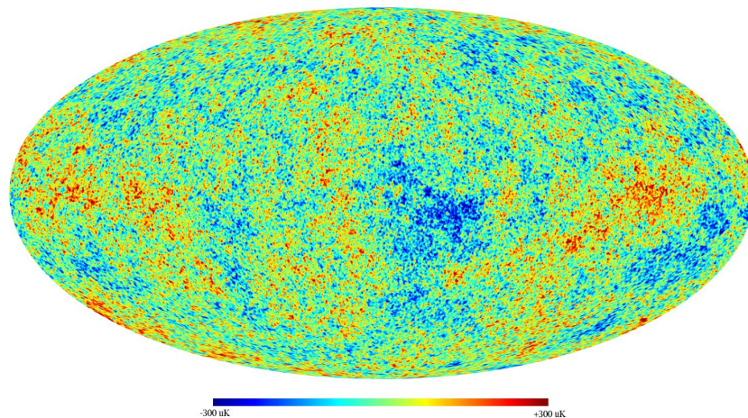
Figura 1.3: Radiación cósmica de fondo. Tomado de http://upload.wikimedia.org/wikipedia/commons/3/3c/Ilc_9yr_moll4096.png
