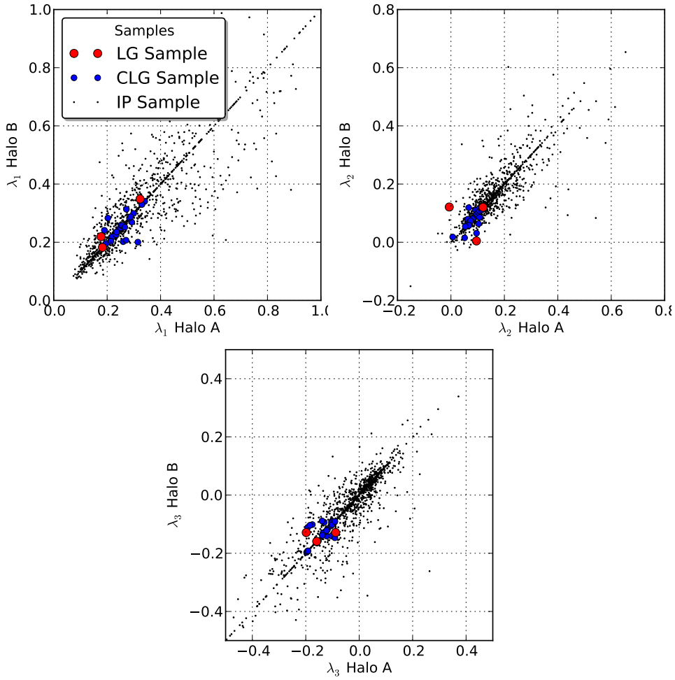
Figura 4.7: Comparación entre las distribuciones de los autovalores de la V-web para los dos halos en los sistemas de pares (muestras LG , CLG y IP ).
