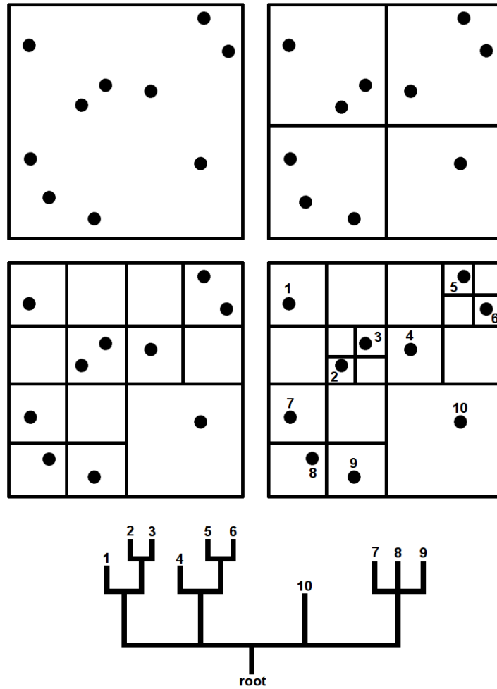
Figura 3.4: Ejemplo de construcción de un código de árbol para una simulación de N-cuerpos. En los paneles superiores se muestran iteraciones del método para un problema 2D. En la parte inferior se ilustra el árbol construido con cada partícula de la simulación.
