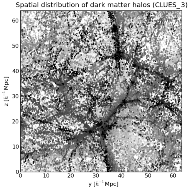
Figura 4.1: Distribución espacial de los halos de materia oscura, reflejando la estructura de la red cósmica. El gradiente de color indica la profundidad respecto al eje x , donde los halos negros son los más cercanos.
