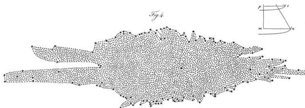
Figura 1.1: Modelo de William Herschel para nuestra galaxia, basado en un conteo de estrellas y la asunción de igual luminosidad [14].
