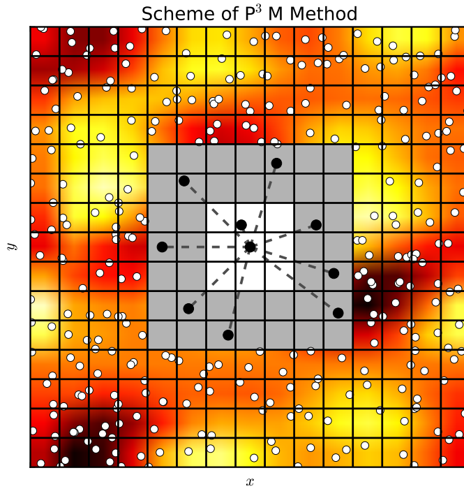
Figura 3.3: Diagrama ilustrativo del método P^3M . Para la partícula de referencia en el centro la interacción con partículas lejanas es calculada con el método PM, mientras que para las partículas cercanas en la región gris y blanca es usado el método de suma directa PP.
