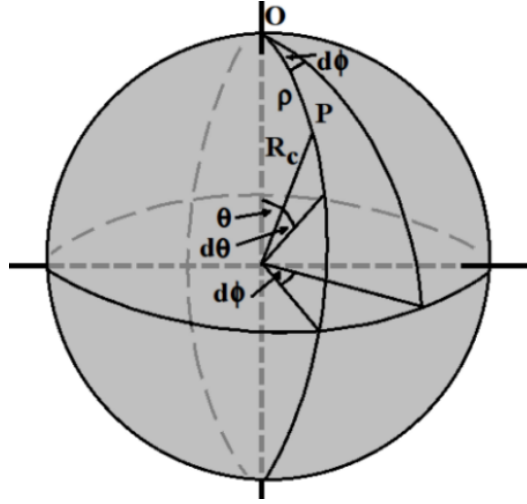
Figura 2.1: Métrica de una superficie esférica.
