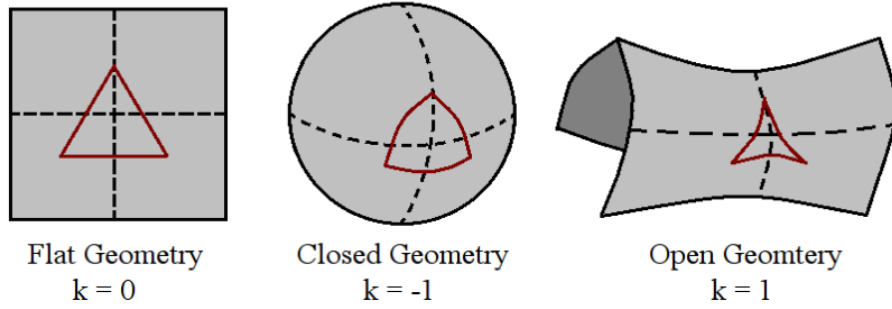
Figura 2.2: Diferentes espacios curvos según el parámetro de curvatura.
