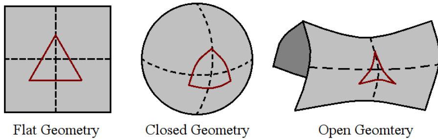
Figura 1.2: Diferentes geometrías con variación del quinto postulado de Euclides.
