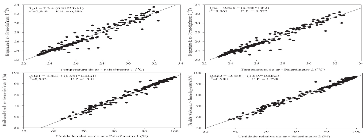
Figura 2 – Correlação entre valores de temperatura obtidos, por meio de psicrômetro aspirado de termopar e um termohigrômetro
