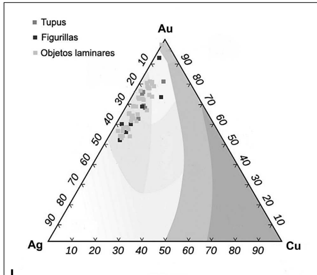
Figura 17 – Diagrama ternario de las aleaciones de oro de los objetos incaicos del Museo de América, con especial referencia al color
